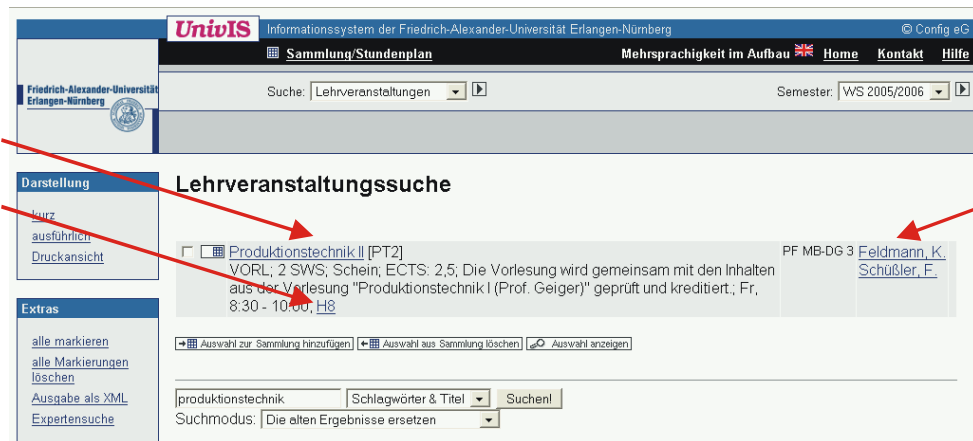
Bild 11: Lehrveranstaltungssuche
